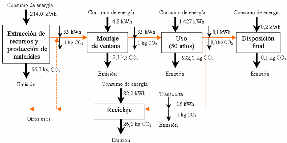
Figura 5.2 Estimación del consumo de energía y emisiones de CO 2 debido a la producción, uso, reciclaje y disposición final de residuos de una ventana de PVC con acristalamiento doble (Uso de un 30% de PVC reciclado en el perfil de la ventana)
